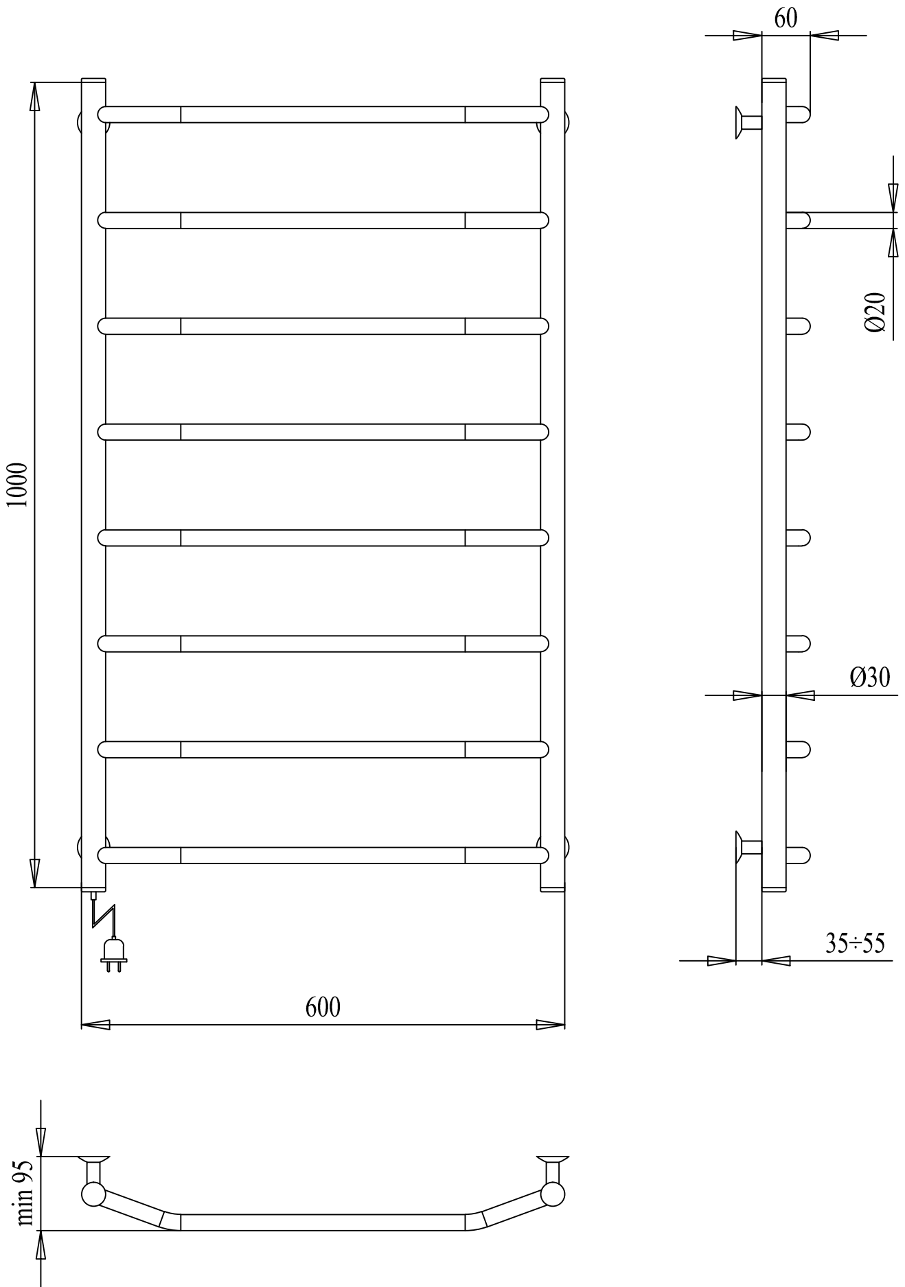
PALADII Рушникосушарка "КЛАСІК ЕЛЕКТРО" 1000x600/8 регулятор L арт. ПШe126PL
