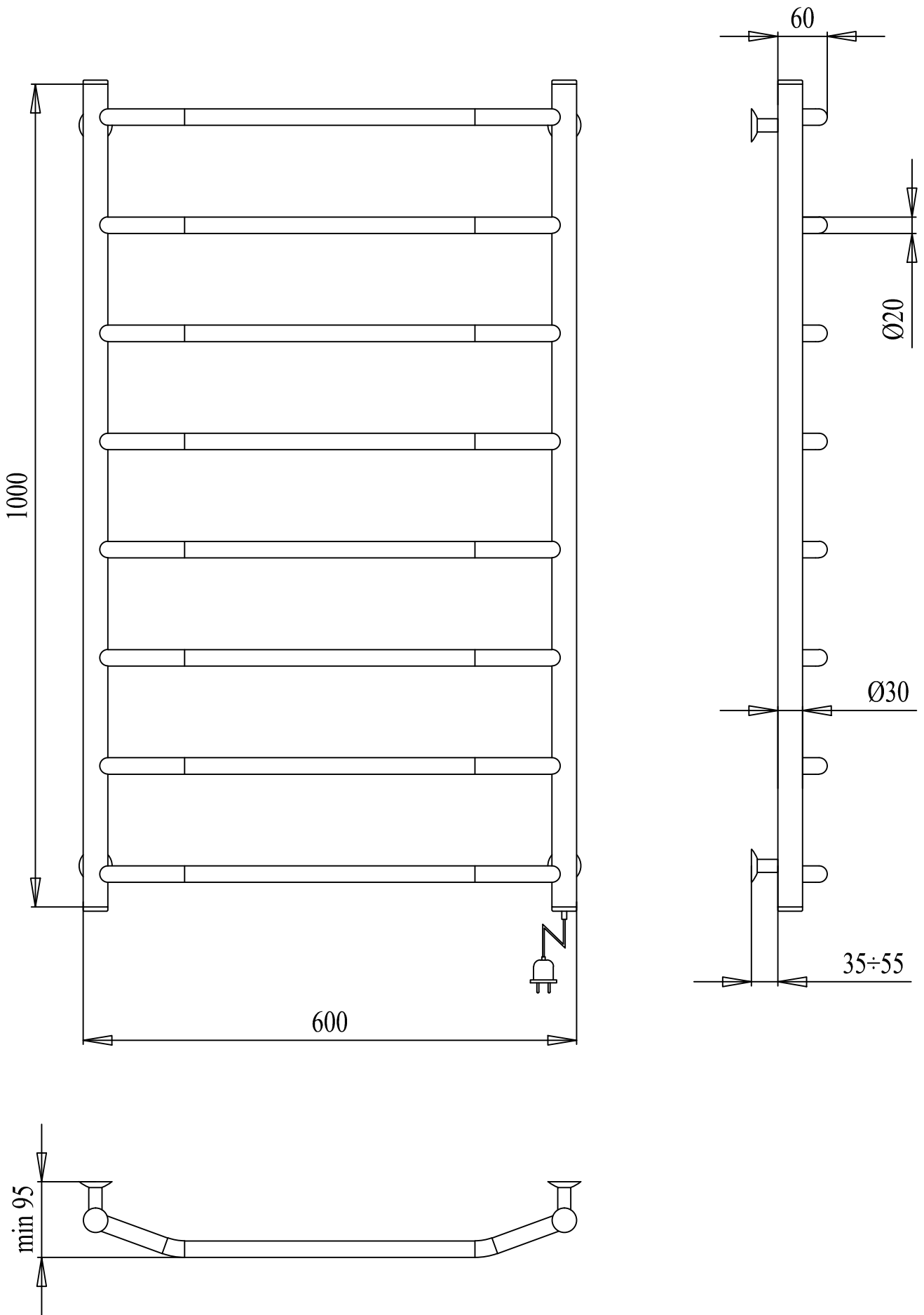
PALADII Рушникосушарка "КЛАСІК ЕЛЕКТРО" 1000х600/8 регулятор R арт. ПШe126PR
