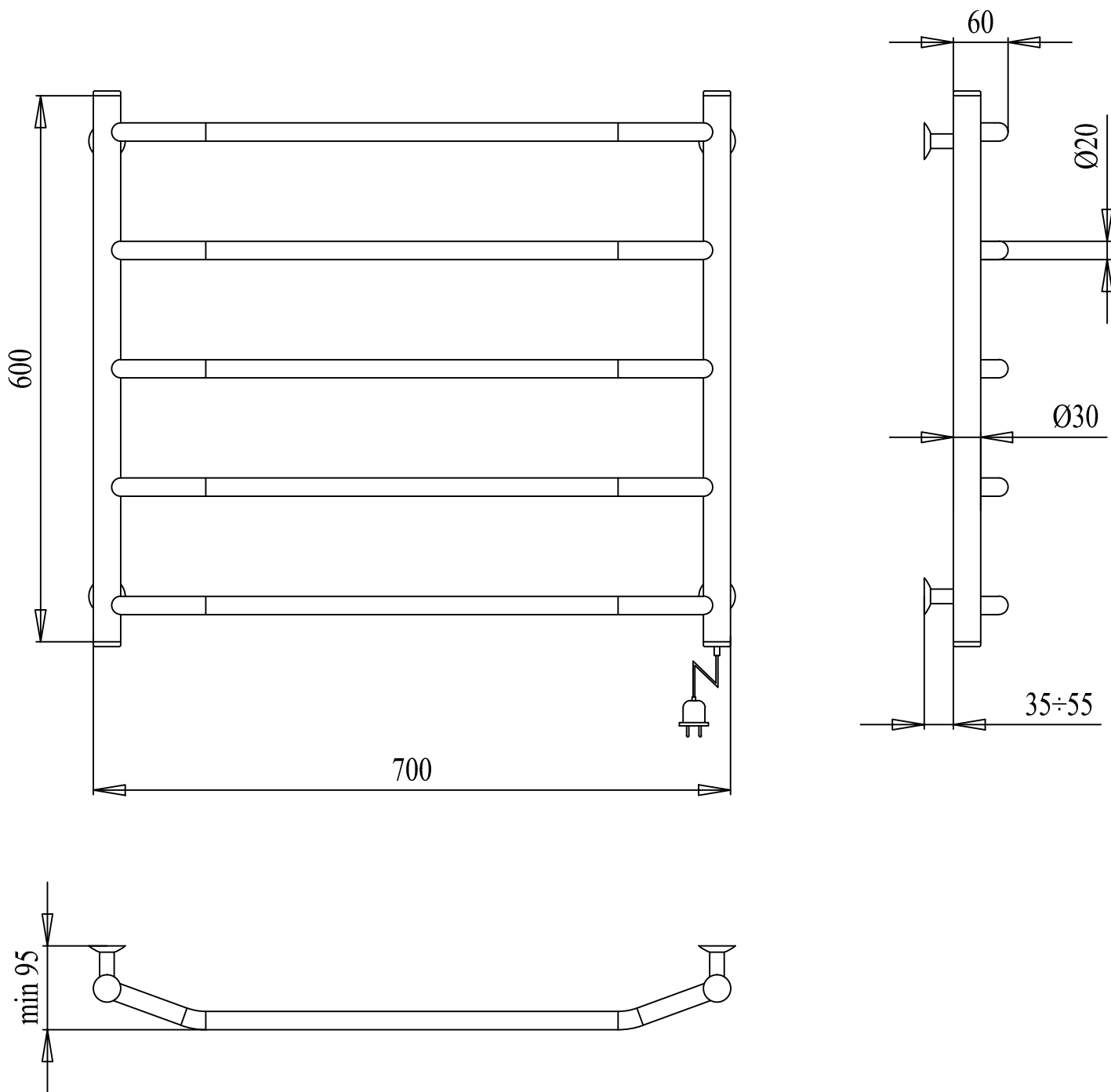
PALADII Рушникосушарка "КЛАСІК ЕЛЕКТРО" 600x700/5 регулятор R арт. PШe101PR
