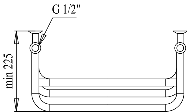
PALADII Рушникосушарка "ОМЕГА" 900x430/7 4м 1/2 арт. ОП013
