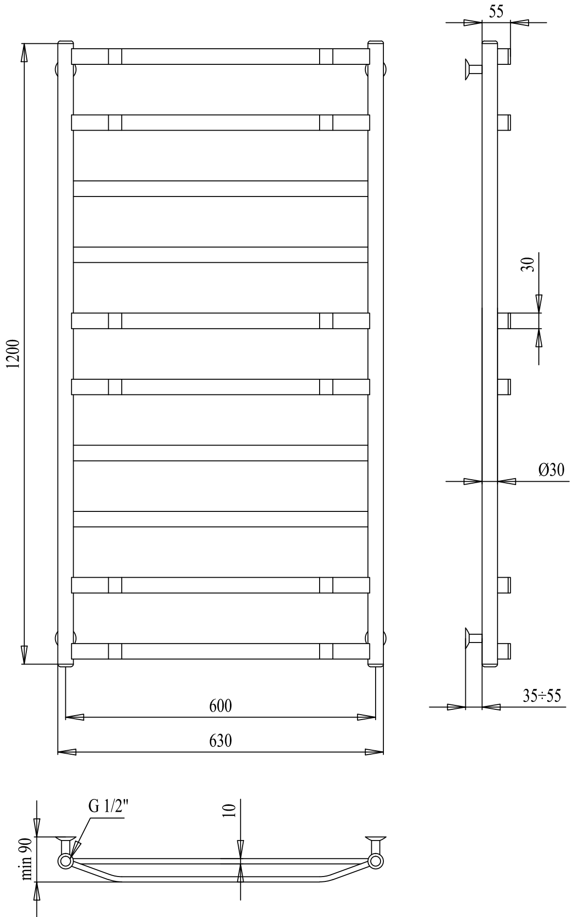
PALADII Рушникосушарка "РИТМ" 1200x630/10 (2+2+2+2+2) 4м 1/2 арт. ПН027
