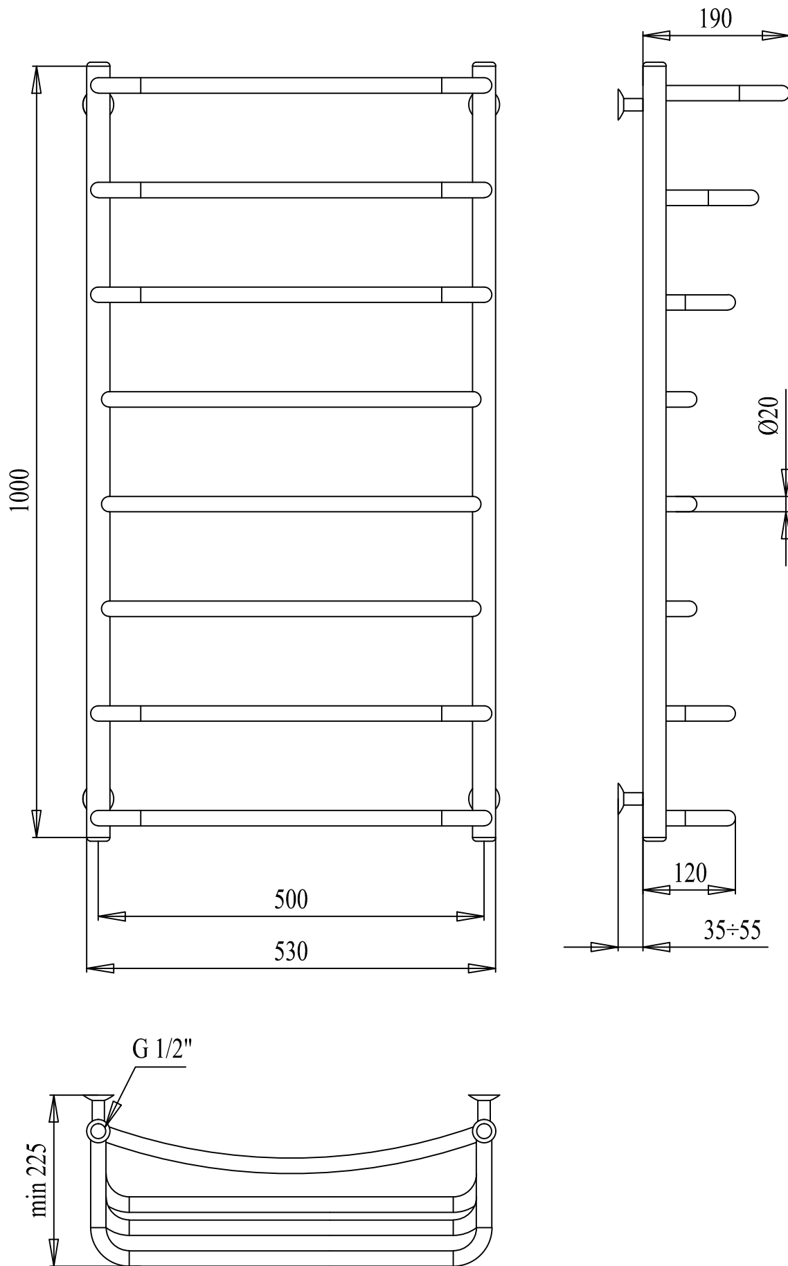
PALADII Рушникосушарка "ТРИУМФ" 1000x530/8 (3п+3+2п) 4м 1/2 арт. ТД003
