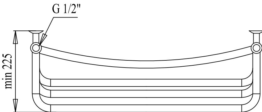
PALADII Рушникосушарка "ТРИУМФ" 900x630/7 (3П+2+2П) 4М 1/2 арт. ТД017
