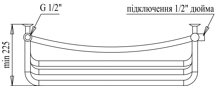
PALADII Рушникосушарка "ТРИУМФ" 900x650/7 (3п+2+2п) 2м 1/2 R арт. ТД116
