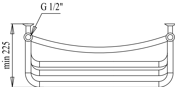
PALADII Рушникосушарка "ТРИУМФ" 900x530/7 (3п+2+2п) 4м 1/2 арт. ТД022
