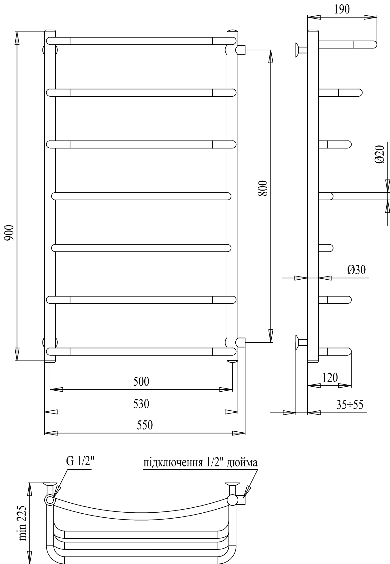
PALADII Рушникосушарка "ТРИУМФ" 900x550/7 (3П+2+2П) 2М 1/2 R арт. ТД114
