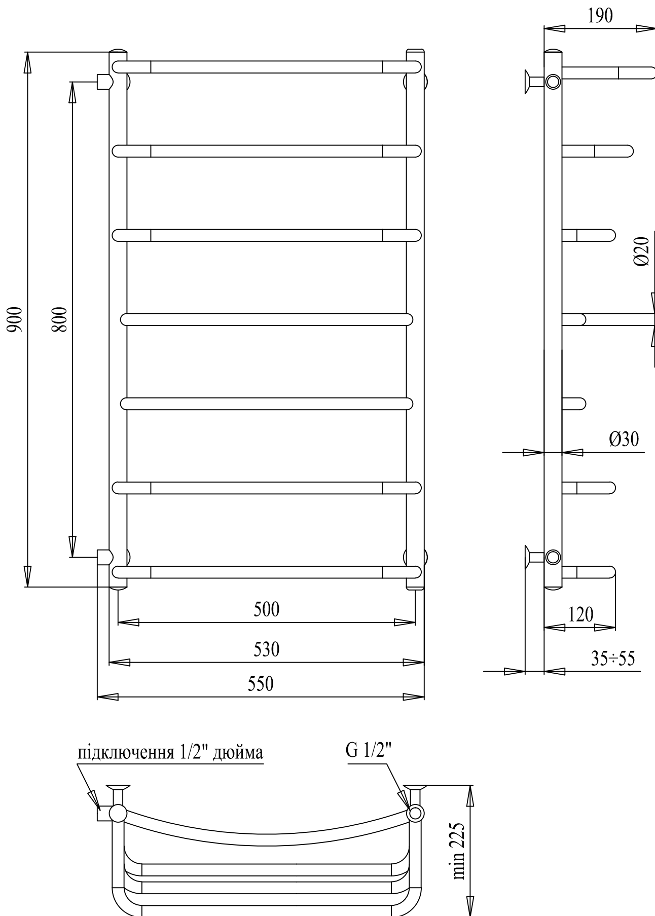
PALADII Рушникосушарка "ТРИУМФ" 900x550/7 (3п+2+2п) 2м 1/2 L арт. ТД108
