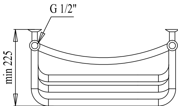
PALADII Рушникосушарка "ТРИУМФ" 900x430/7 (3п+2+2п) 4м 1/2 арт. ТД021
