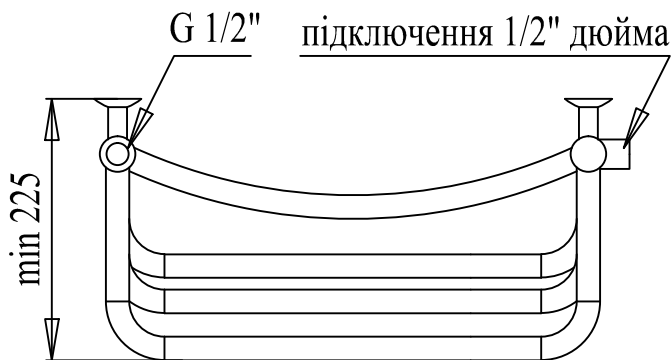
PALADII Рушникосушарка "ТРИУМФ" 900x450/7 (3п+2+2п) 2м 1/2 R арт. ТД113
