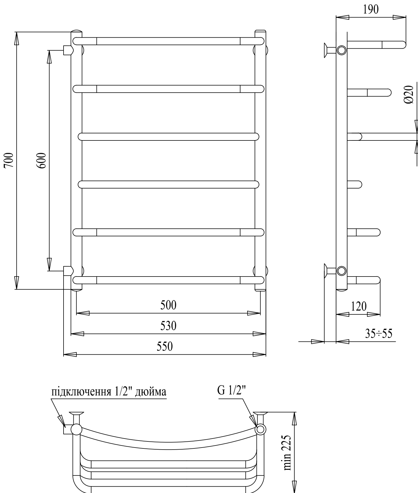
PALADII Рушникосушарка "ТРИУМФ" 700x550/6 (2п+2+2п) 2м 1/2 L арт. ТД111
