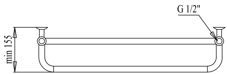
PALADII Рушникосушарка "УНІВЕРСАЛ" 1200x630/12 (1+1п+2+1п+2+1п+2+1п+1) 4м 1/2 арт. УР010
