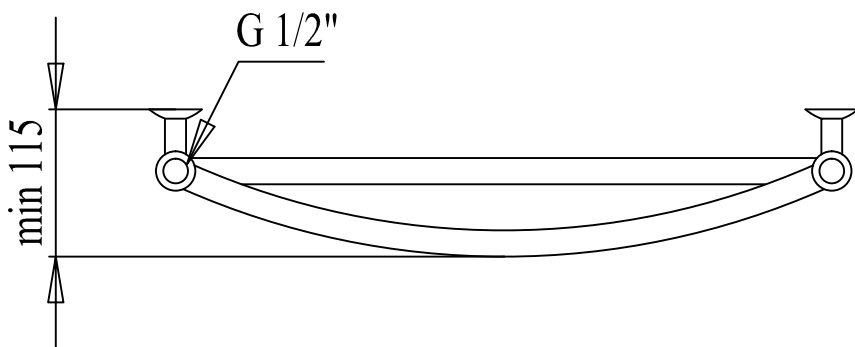
PALADII Рушникосушарка "МІКС" 850x530/7 (2+3пр+2) 4м 1/2 арт. СП002
