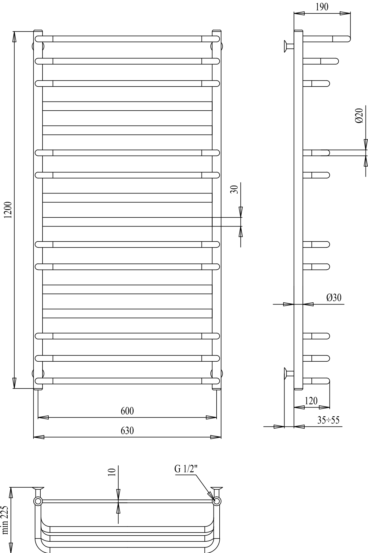
PALADII Рушникосушарка "ТРИО" 1200x630/16(3+2П+2+2П+2+2П+3)4М 1/2 арт. УТ005
