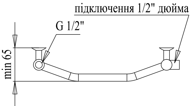
PALADII Рушникосушарка "КЛАСІК" 550x400/5 2м 1/2 арт. РШ085
