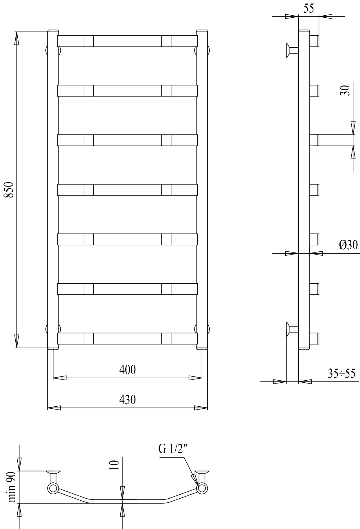
PALADII Рушникосушарка "ГАЛАНТ" 850x430/7 4м 1/2 арт. ПТ020
