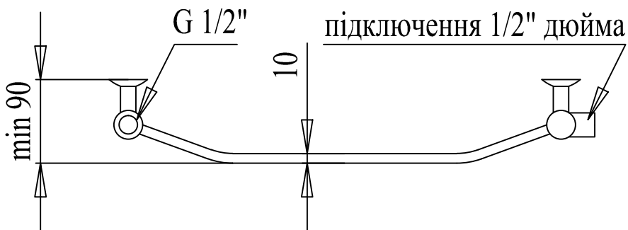
PALADII Рушникосушарка "ГАЛАНТ" 650x500/5 2м 1/2 арт. ПТ033
