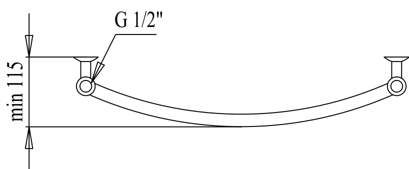
PALADII Рушникосушарка "СТАНДАРТ" 550x530/5 4м 1/2 арт. РБ028
